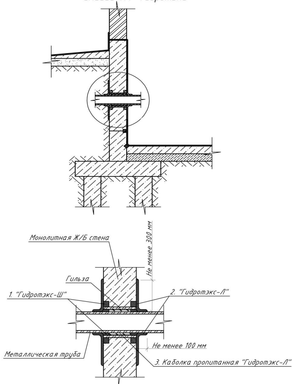
Рисунок 5: Устройство гидроизоляции вводов коммуникаций, с применением сухих дисперсных строительных гидроизоляционных проникающих капиллярных смесей ТМ «Гидротэкс»
